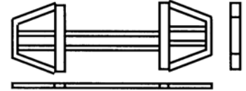
Četrax cisternas rāmis
