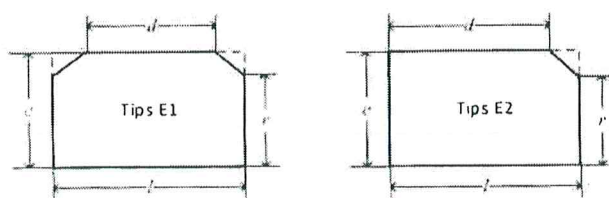
1. att. Koka pārmiju brusu un gulšņu šķērsgriezumu tipi
