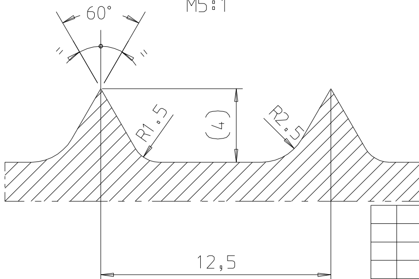
Detāļa A M5:1
