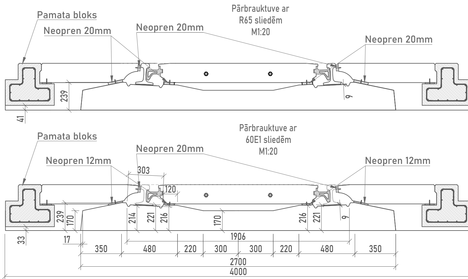
Stiegru novietojums. Griezums A-A M1:20
