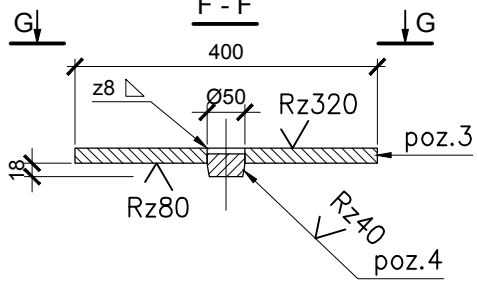
Aukšējais balansieris
