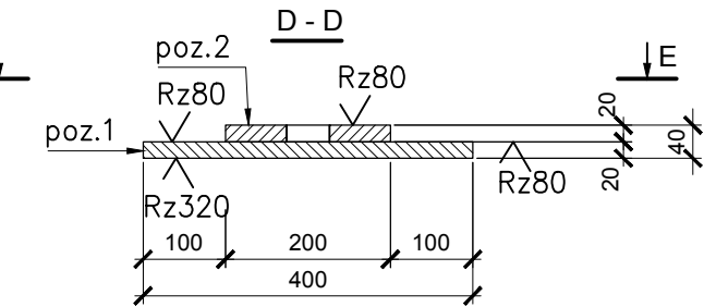
Apakšējais balansieris
