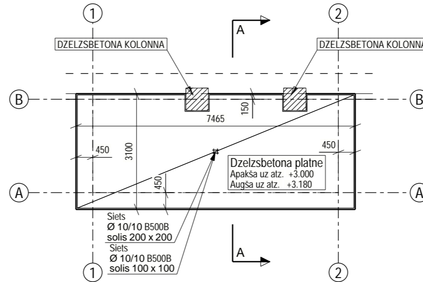
Pagrabstava parseguma plans 1:100
