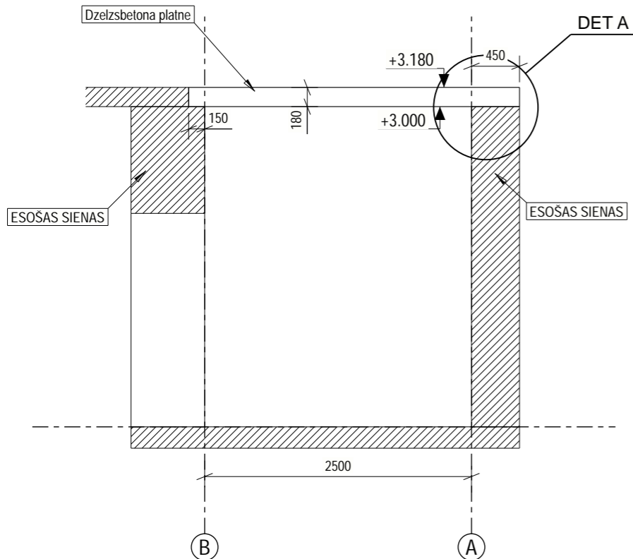
A - A 1:50
