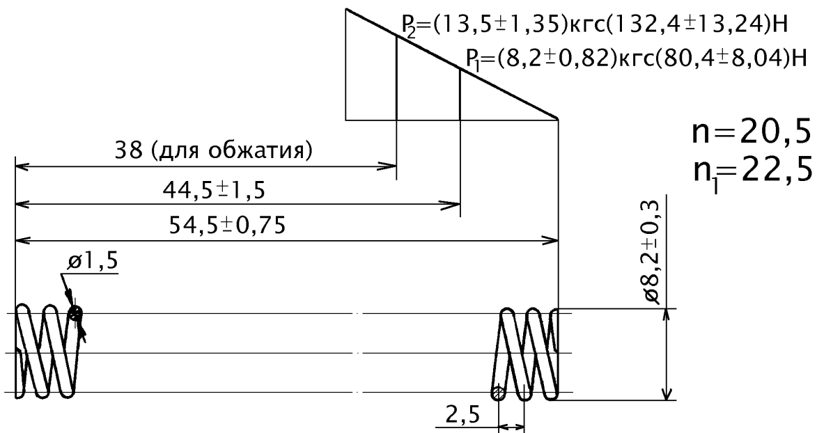
Рисунок 38 - Пружина 270.605-1
