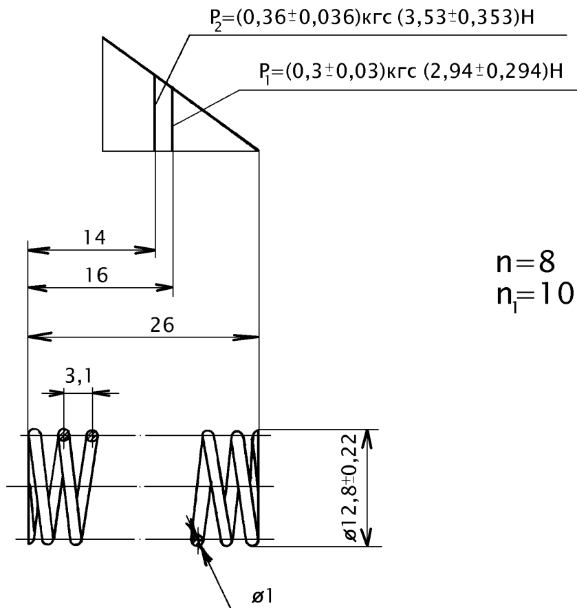
Рисунок 36 - Пружина 87.02.21
