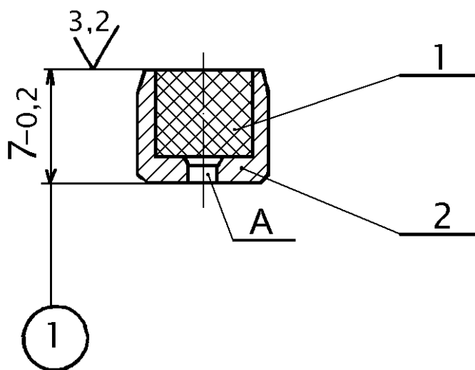
Рисунок 23 – клапан 483.110
