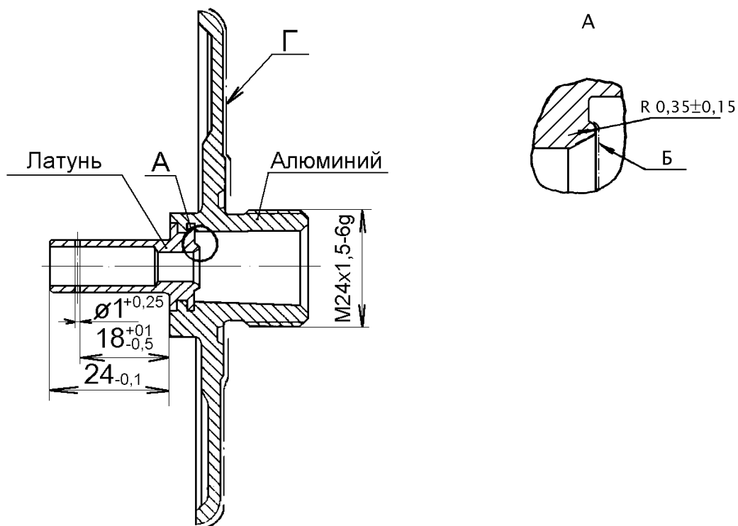
Рисунок 14 - Диск направляющий P483.014
