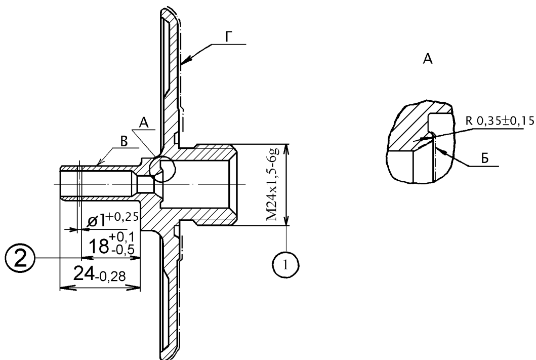
Рисунок 13 – Диск направляющий 483.014
