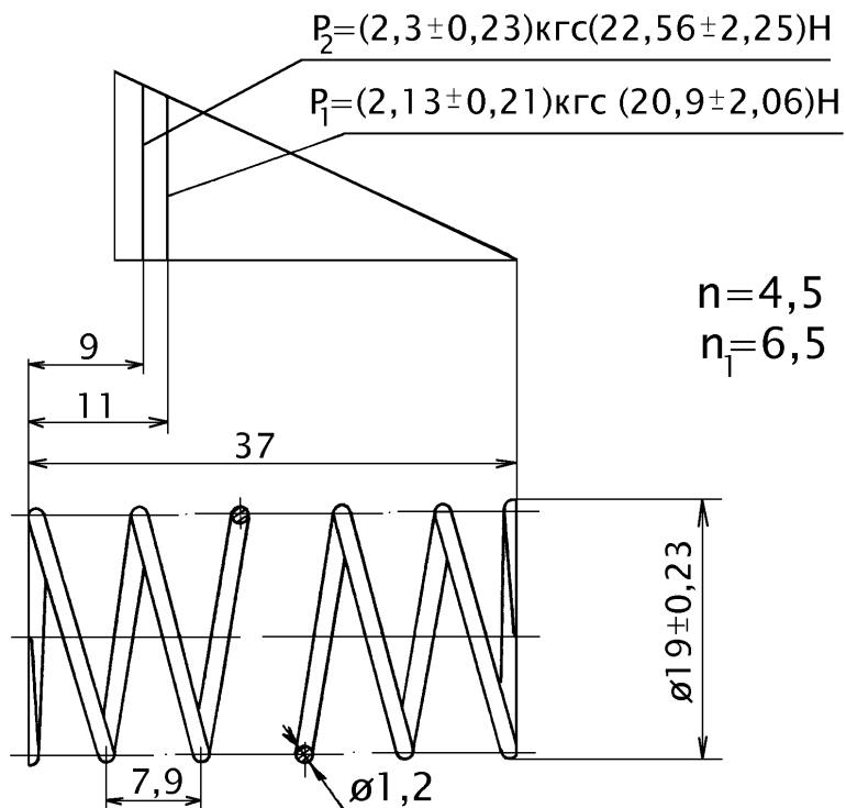
Рисунок 32 - Пружина 483.002
