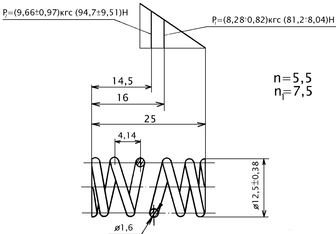
Рисунок 34 - Пружина 483.031
