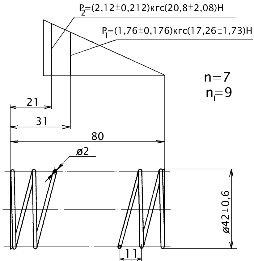
Рисунок 35 - Пружина 483.004
