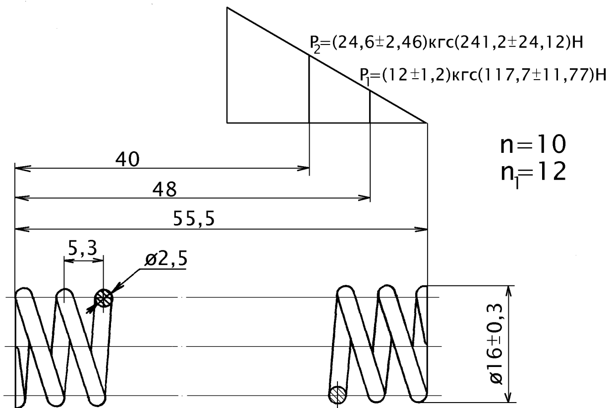
Рисунок 39 - Пружина 270.371
