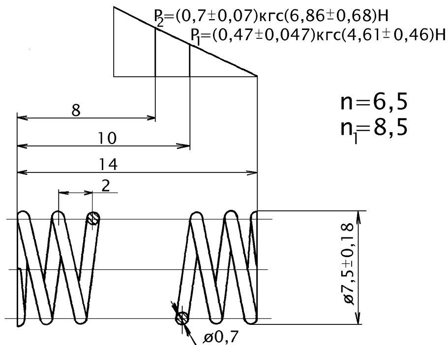
Рисунок 37 - Пружина 305.108
