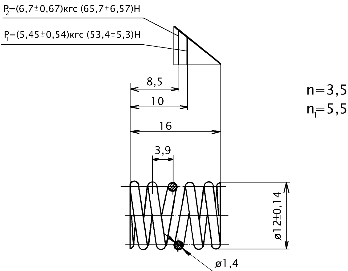
Рисунок 33 - Пружина 483.029
