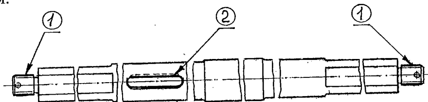
Рисунок 5.176 – Вал
