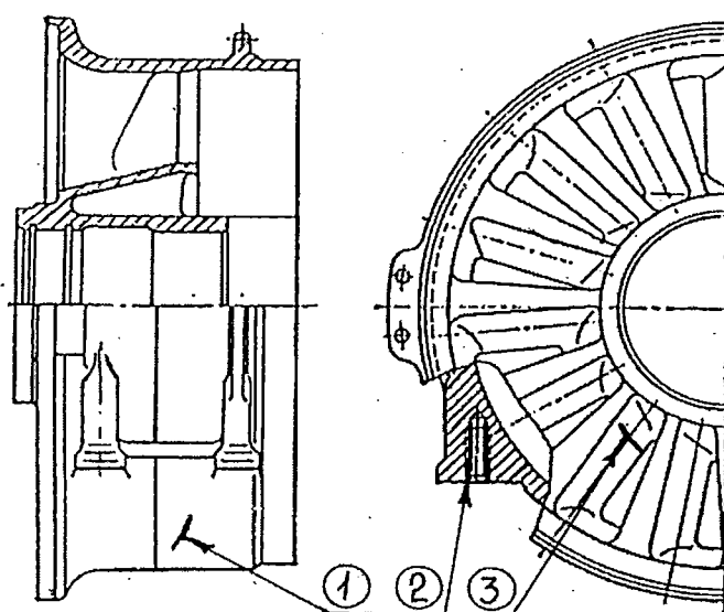
Рисунок 5.96 – Устройство воздухонаправляющее
