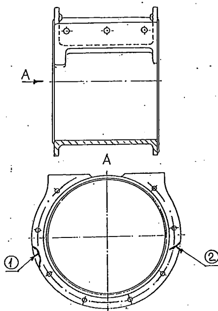
Рисунок 5.26 - Корпус тормозного цилиндра
