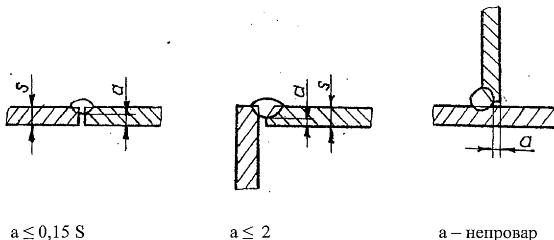
Рисунок 3.1 - Допустимая величина непровара
