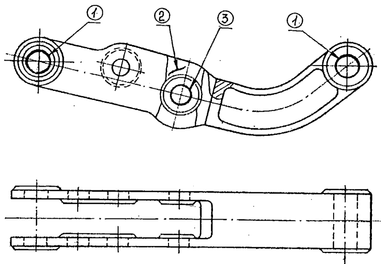
Рисунок 5.179 – Рычаг
