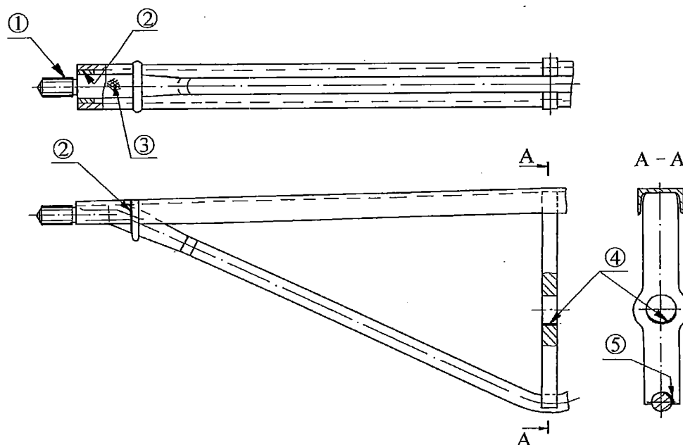
Рисунок 5.29 - Балка триангеля со струной и распоркой
