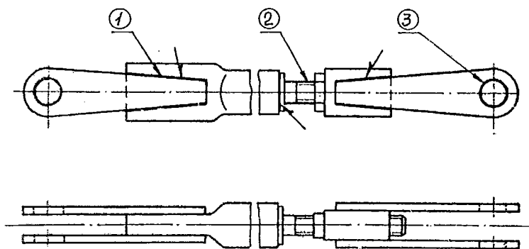
Рисунок 5.169 - Тяга
