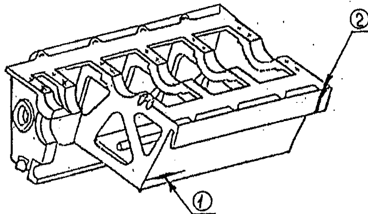
Рисунок 5.89–Картер коленчатого вала
