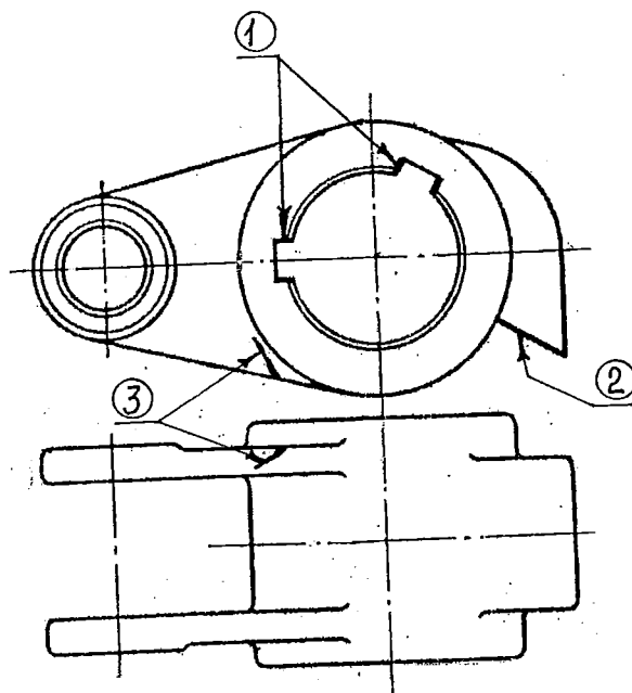
Рисунок 5.175 - Рычаг поворотный
