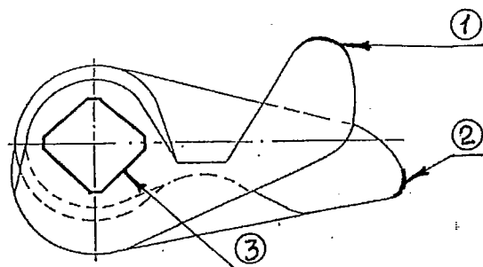
Рисунок 5.45 – Подъемник замка
