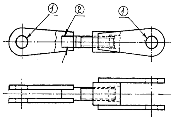
Рисунок 5.171 - Тяга
