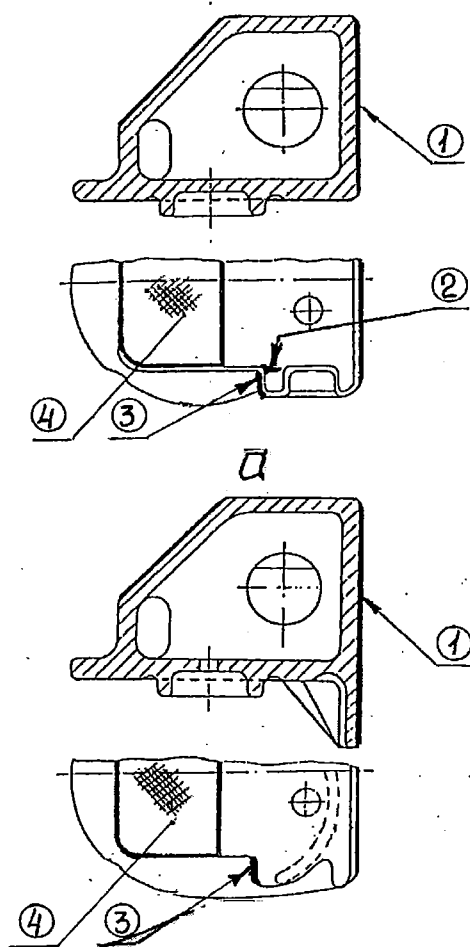
Рисунок 5.9 – Клин а - чертеж 100.30.001-0; б – чертеж 100.30.001-1
