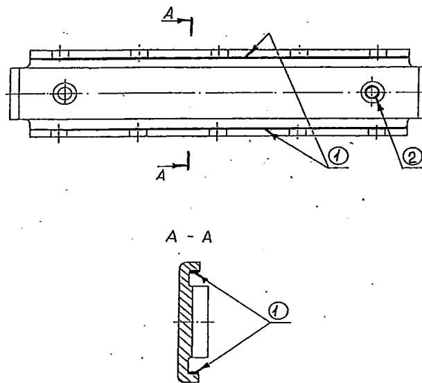
Рисунок 5.23 – Планка рессорная
