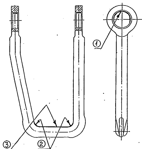
Рисунок 5.32 – Подвеска триангеля
