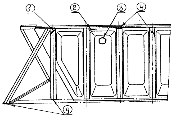
Рисунок 5.149 - Кузов
