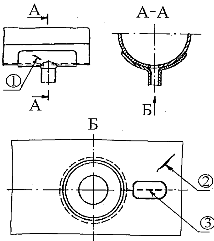
Рисунок 5.132 - Броневой лист
