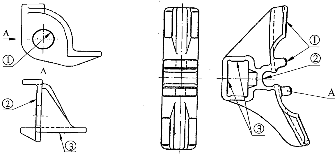
Рисунок 5.30 - Наконечник триангеля Рисунок 5.31 - Башмак неповоротный
