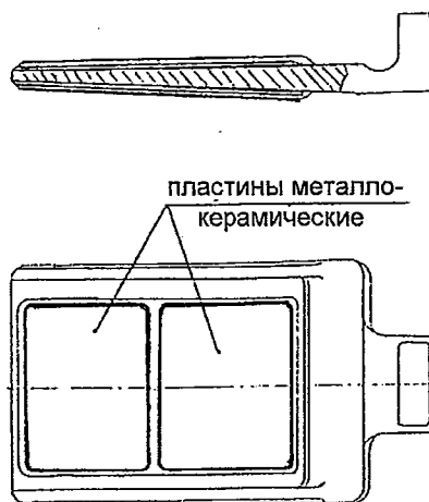
Рисунок 5.55 - Пласти́на неподвижная
