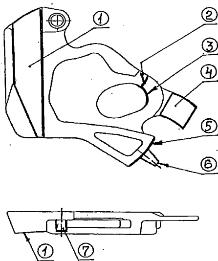
Рисунок 5.42 – Замок
