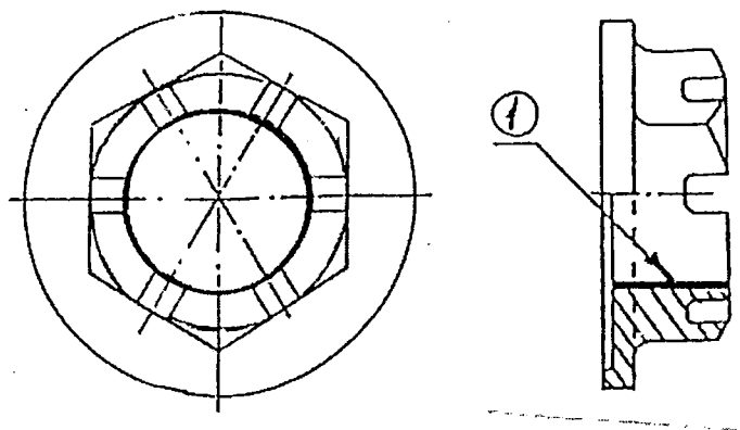
Рисунок 7.14 – Гайка шпинтона
