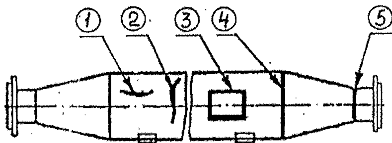
Рисунок 5.93 - Глушитель
