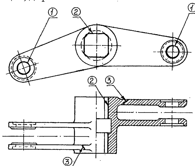
Рисунок 5.178— Вилка поворотная
