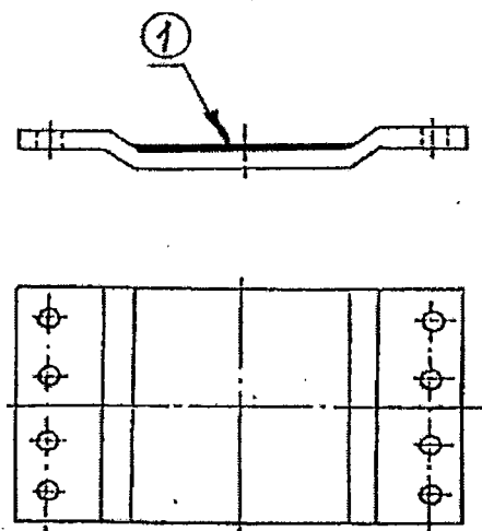
Рисунок 5.60 – Планка поддерживающая
