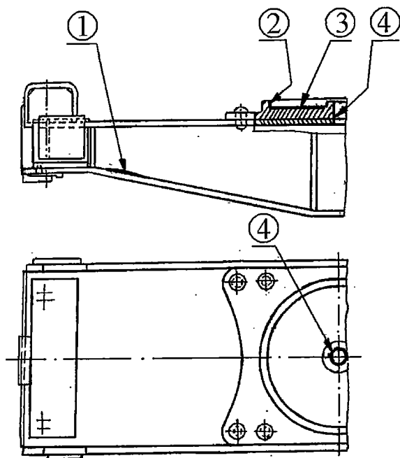
Рисунок 5.17 - Брус наддрессорный
