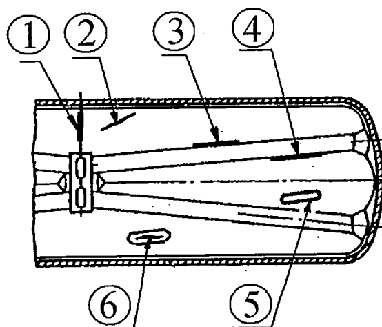
Рисунок 5.145 - Устройство аэропневмовыгрузки
