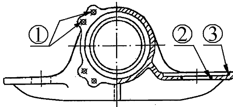
Рисунок 5.11 - Корпус буксы
