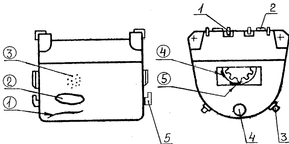
Рисунок 5.147 – Бункер 1 – петля; 2 – ручка; 3 – штупцер; 4 – подушка; 5 – упор
