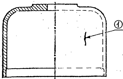
Рисунок 5.115 – Крышка внутренняя масляной центрифуги
