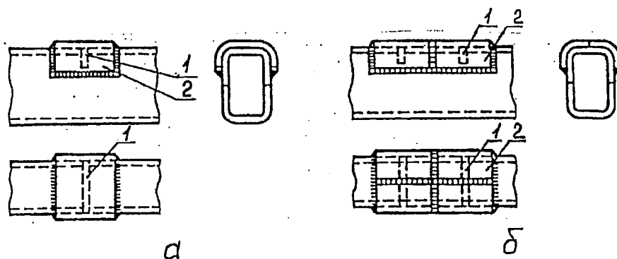
Рисунок 3.3 - Схемы конструктивных усиления после заварки трещин:
