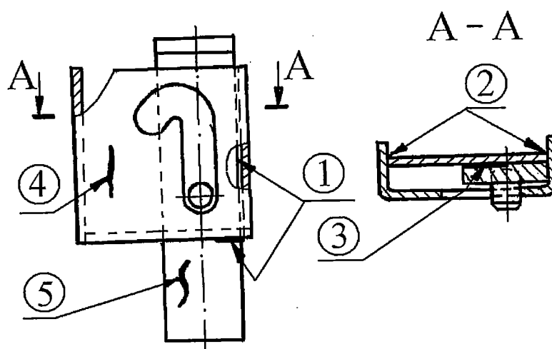
Рисунок 5.87 - Нижний запорный механизм торцевой двери полувагона
