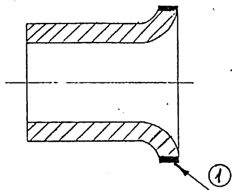
Рисунок 5.40 Втулка упорная регулятора 74 Б
