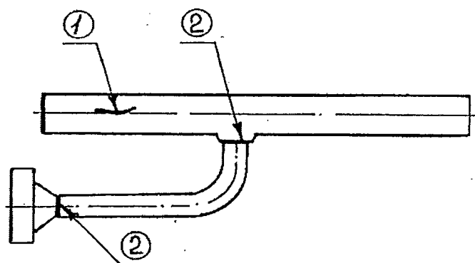
Рисунок 5.112 - Подвод
