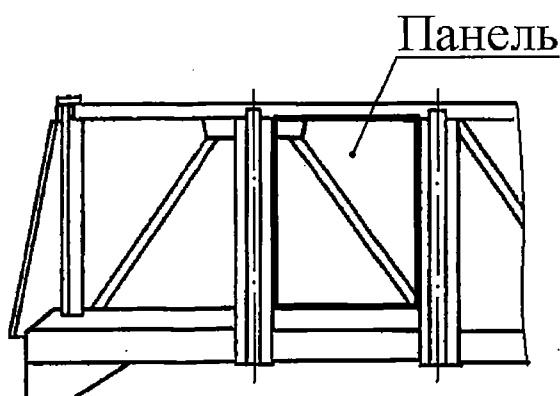
Рисунок 5.78 – Обшивка вагона
