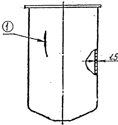
Рисунок 5.103 – Стакан топливного фильтра
