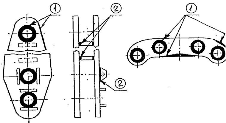
Рисунок 5.36 - Рычаги тормозные и затяжки рычагов
