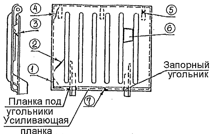
Рисунок 5.83 – Крышка люка полувагона
