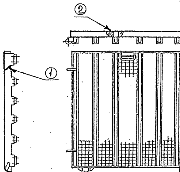
Рисунок 5.128- Решетка напольная
