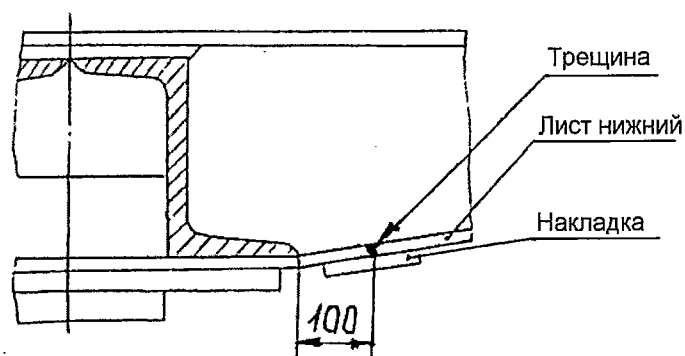
Рисунок 5.70 - Нижний лист шкворневой балки, отремонтированный сваркой
