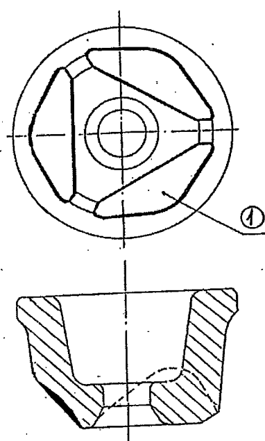
Рисунок 5.53 - Конус нажимной
