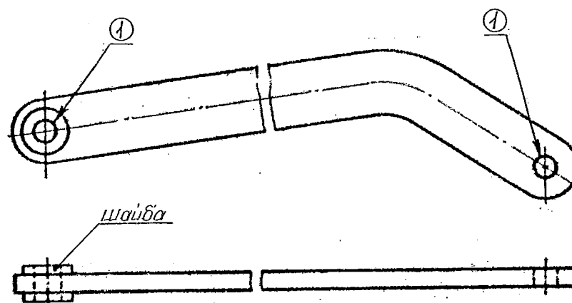
Рисунок 5.163 – Рычаг
