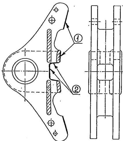
Рисунок 5.34 – Башмак
