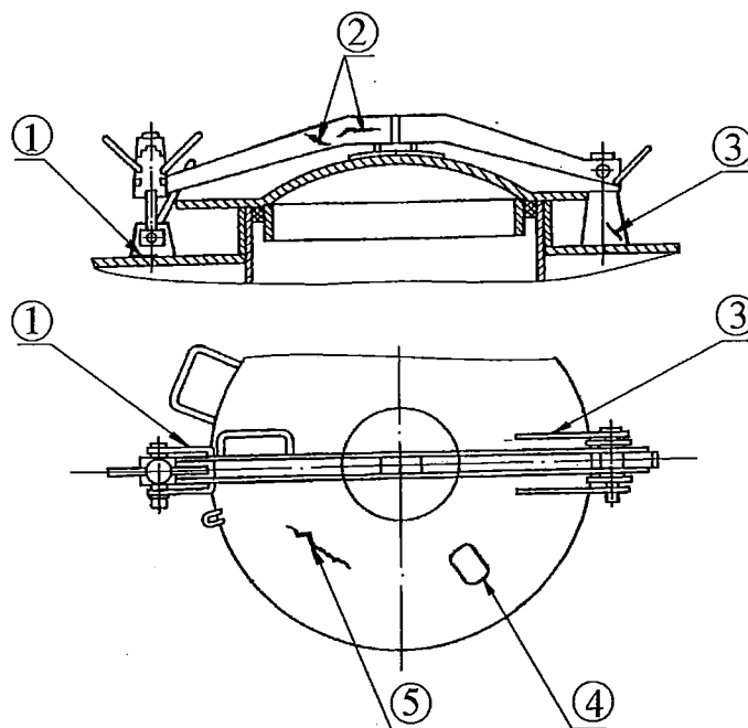
Рисунок 5.136 - Крышка ригельного типа
