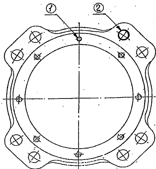
Рисунок 5.12 – Крышка крепительная
