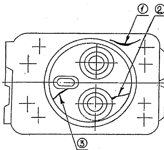
Рисунок 5.90 – Головка цилиндра
