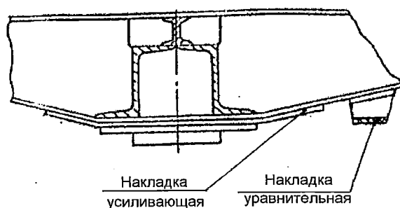
Рисунок 5.71 - Усиление накладкой нижнего листа шкворневой балки полувагона
