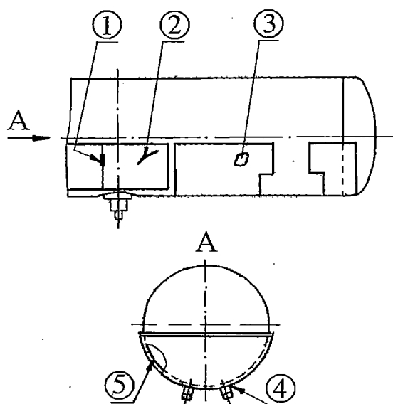
Рисунок 5.142 - Паровая рубашка котла
