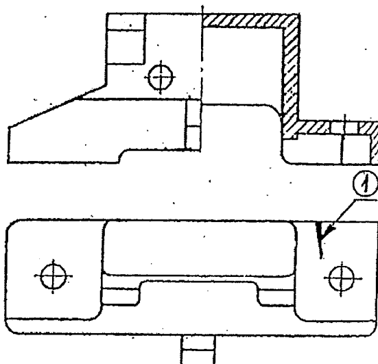
Рисунок 5.125 - Лапа крепления асинхронного двигателя
