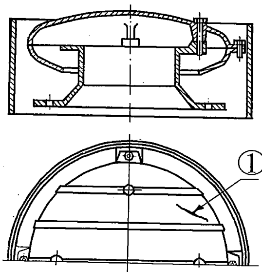
Рисунок 5.126 - Дефлектор
