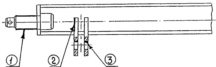
Рисунок 5.33 – Траверса
