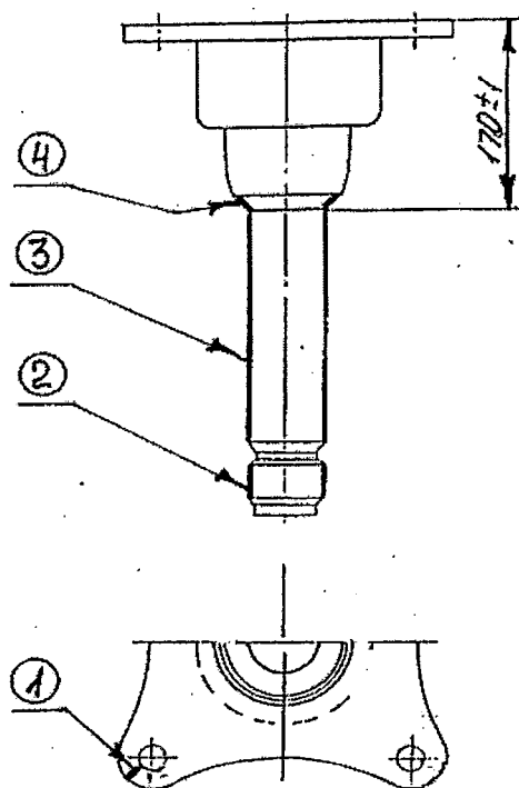
Рисунок 5.13— Шпинтон
