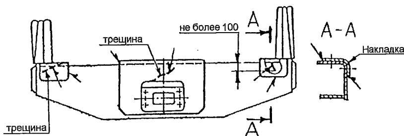
Рисунок 5.67 - Балка полувагона с металлической обшивкой, отремонтированная сваркой
