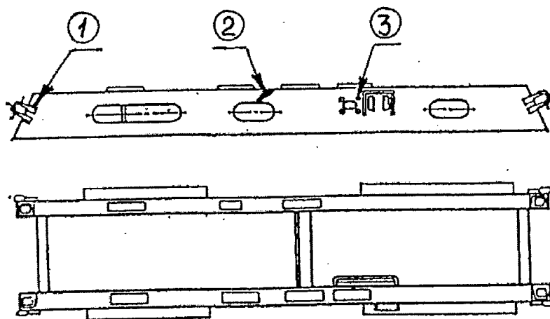
Рисунок 5.109 – Рама дизель – генератора
