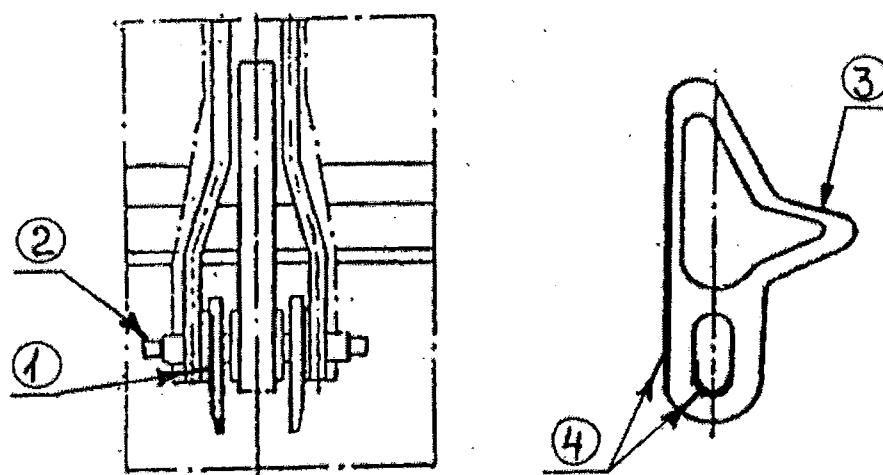
Рисунок 5.86 – Детали запоров бортов платформы
