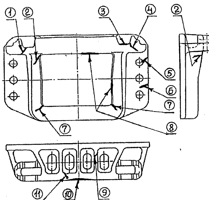
Рисунок 5.47 – Розетка ударная
