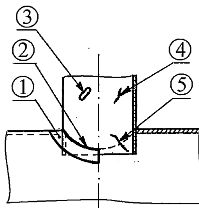
Рисунок 5.134 - Колпак цистерн
