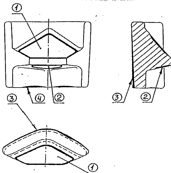
Рисунок 5.54 - Кли́н фрикционный
