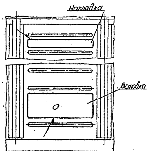
Рисунок 5.81 – Приварка накладки и вставки в межстоечный проем
