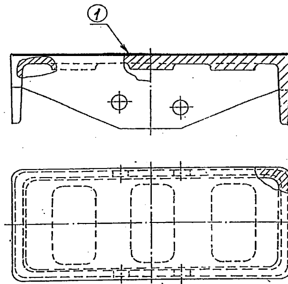
Рисунок 5.10 - Колпак скользуна
