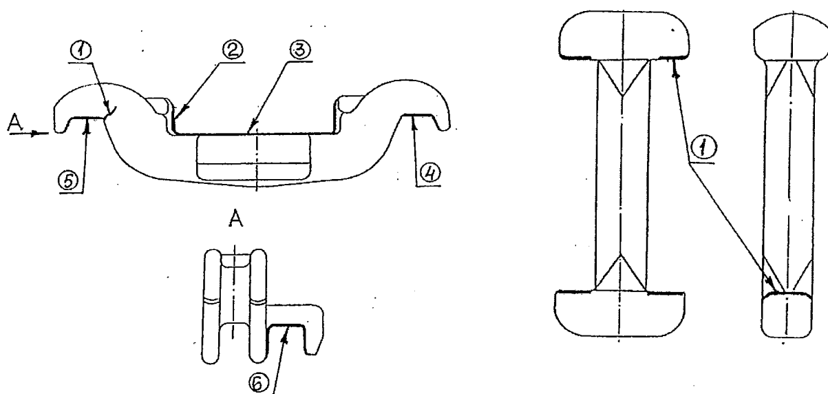
Рисунок 5.49 – Подвеска маятниковая
