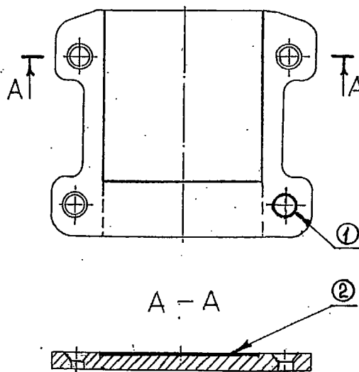
Рисунок 5.8 - Планка фрикционная
