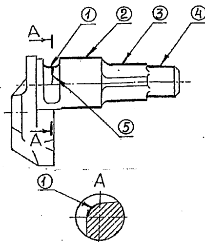
Рисунок 5.46 – Валик подъемника
