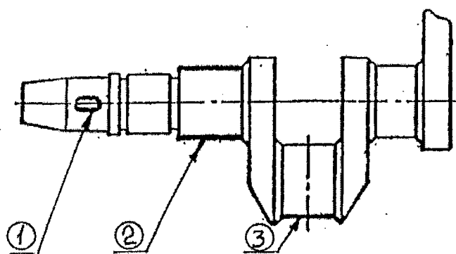
Рисунок 5.91 – Вал коленчатый
