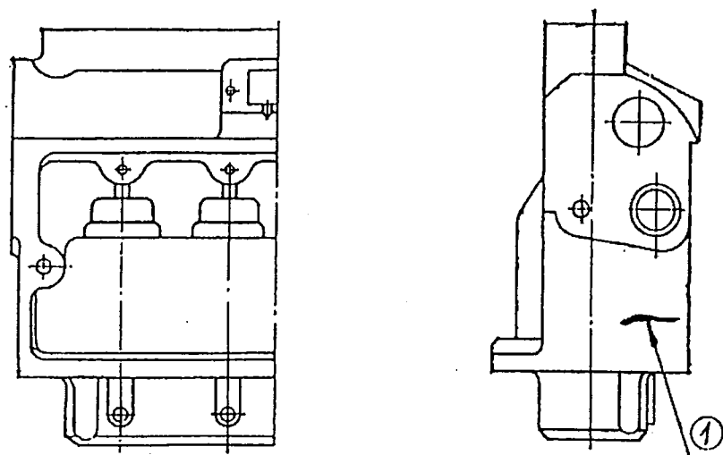
Рисунок 5.99 – Корпус топливного насоса
