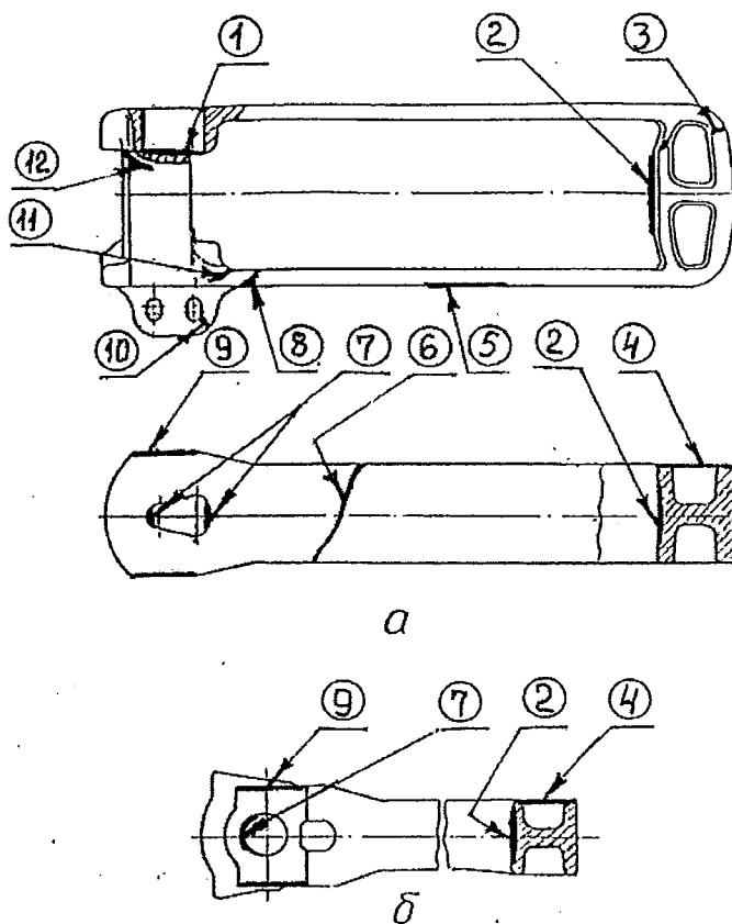
Рисунок 5.57 - Хомут тяговый: а - для автосцепки СА-3; б - для автосцепки СА-3М
