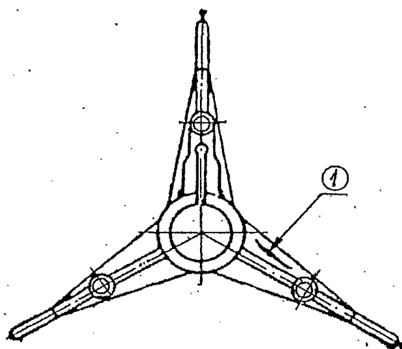
Рисунок 5.124 - Вентилятор асинхронного двигателя
