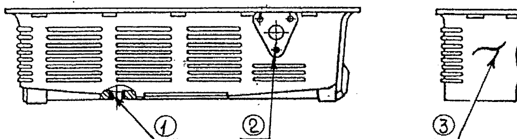
Рисунок 5.95- Ванна масляная
