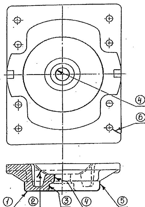
Рисунок 5.73 – Пятник
