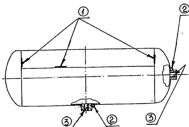
Рисунок 5.25 – Резервуар воздушный
