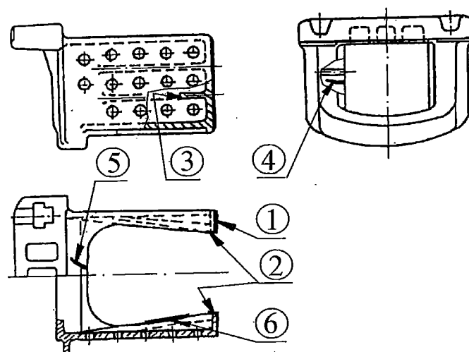
Рисунок 5.58- Упор передний
