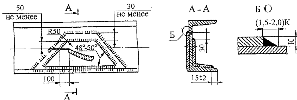
Рисунок 3.4 - Приварка двусторонних накладок со смещением противоположных швов
