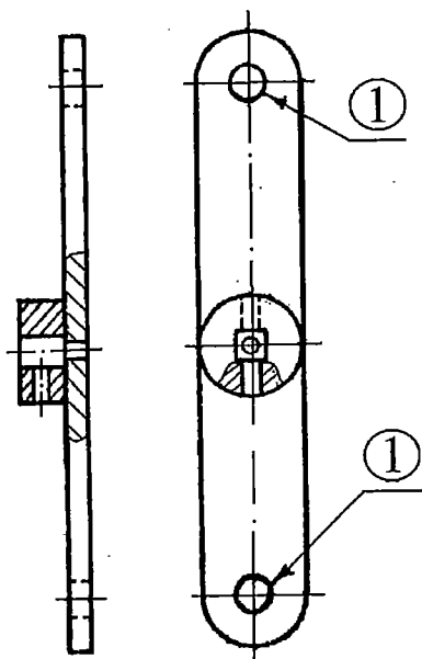
Рисунок 5.172 – Рычаг
