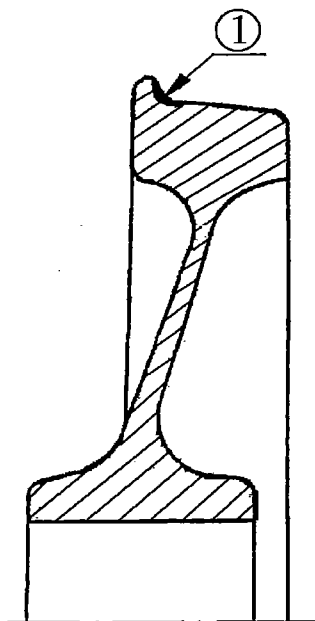
Рисунок 5.2 - Колесо цельнокатаное
