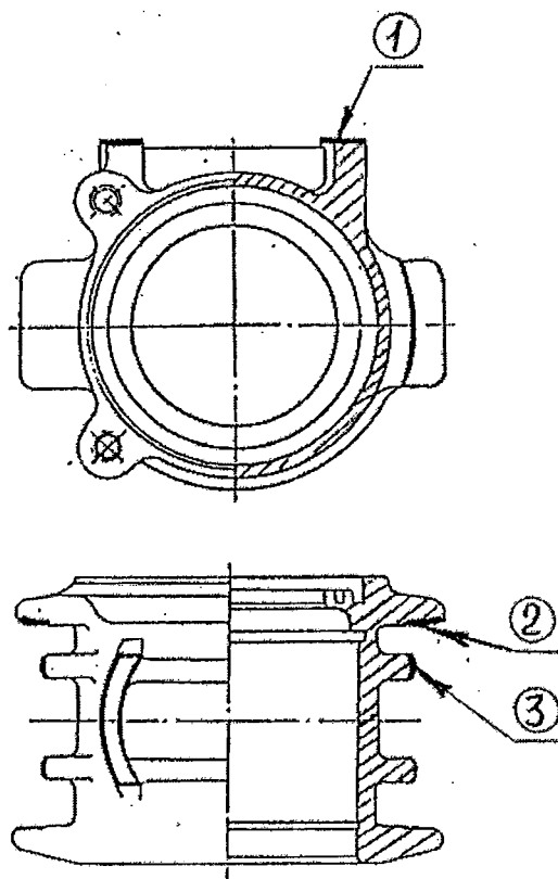
Рисунок 5.4 - Корпус буксы
