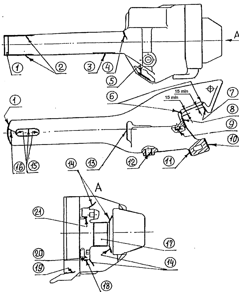
Рисунок 5.41 Корпус автосцепки
