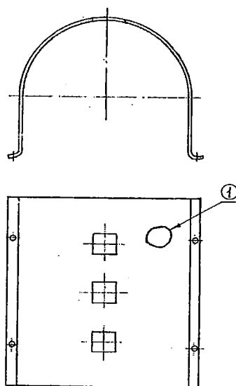
Рисунок 5.180 – Кожух цилиндра
