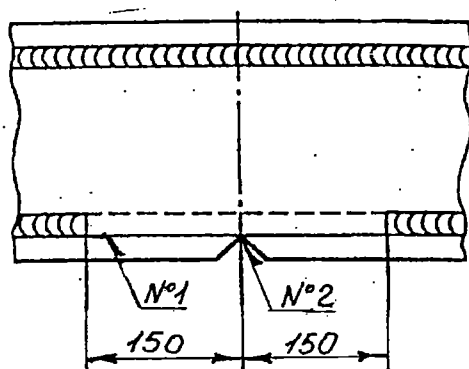
Рисунок 3.2 - Схема подготовки к заварке трещин в элементах типа сварных балок коробчатого сечения
