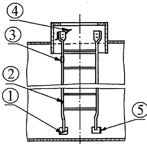
Рисунок 5.140 - Внутренняя лестница
