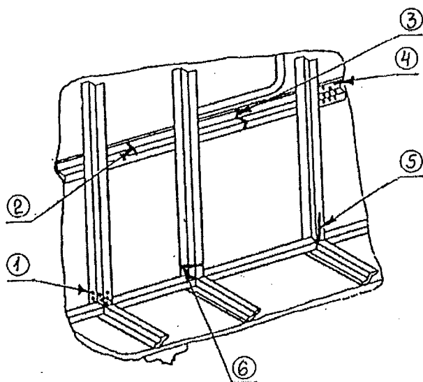
Рисунок 5.76 – Каркас кузова рефрижераторного вагона
