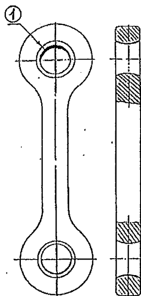
Рисунок 5.21 – Подвеска
