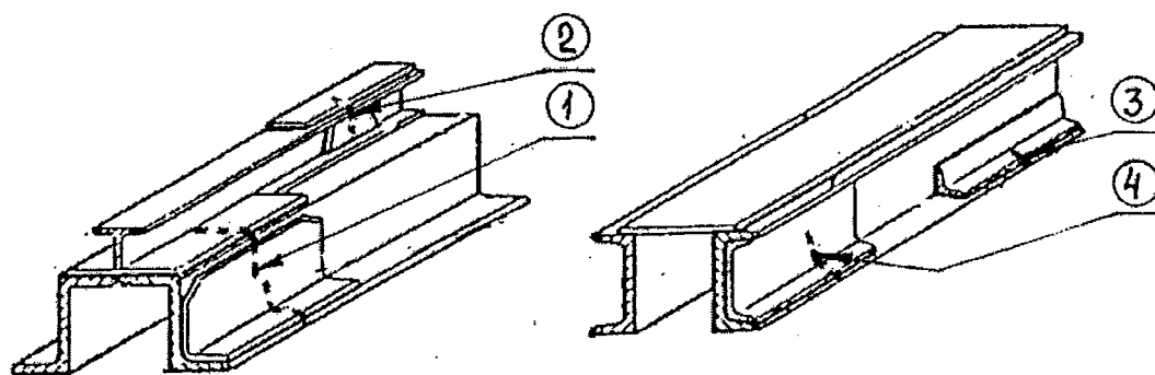
Рисунок 5.62 - Балки хребтовые с трещинами и изломами, отремонтированные накладками
