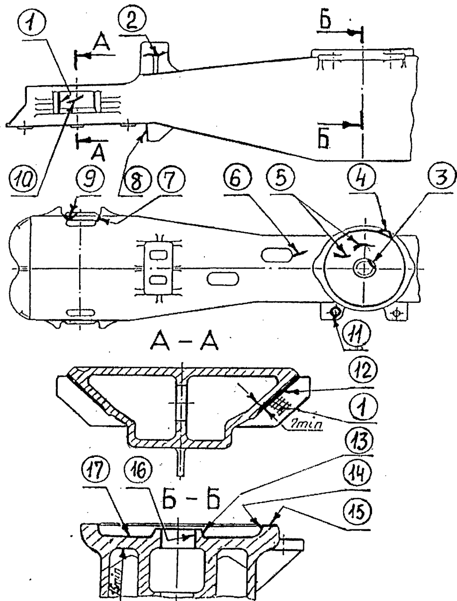
Рисунок 5.5 - Балка надрессорная
