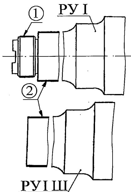
Рисунок 5.1 - Ось
