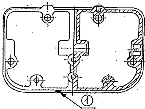
Рисунок 5.113 – Кронштейн коромысла
