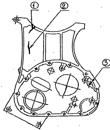
Рисунок 5.104 - Картер шестерен газораспределения
