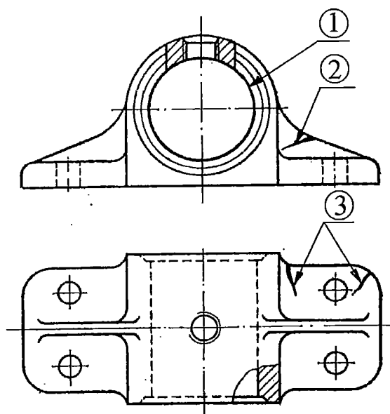
Рисунок 5.174 – Подшипник
