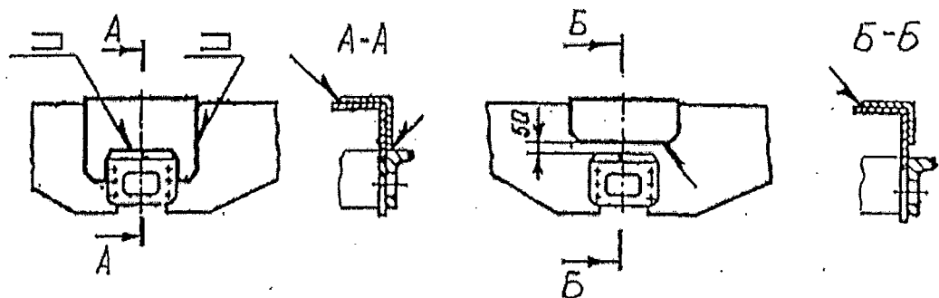
Рисунок 5.64 - Постановка накладки на балке над ударной розеткой
