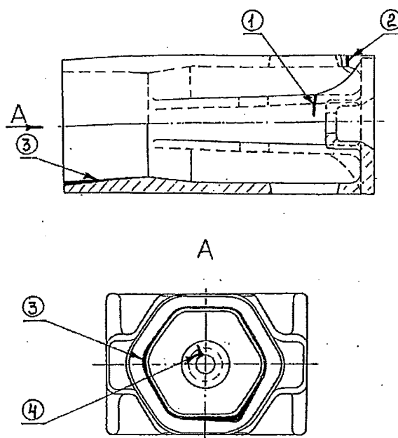
Рисунок 5.52 - Корпус поглощающего аппарата
