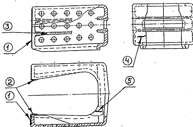
Рисунок 5.59 - Упор задний
