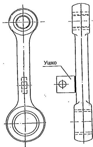
Рисунок 5.35 - Подвеска башмака
