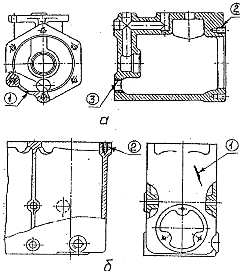
Рисунок 5.94 - Корпус масляного фильтра:
