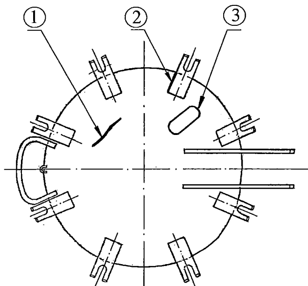
Рисунок 5.135 - Крышка колпака
