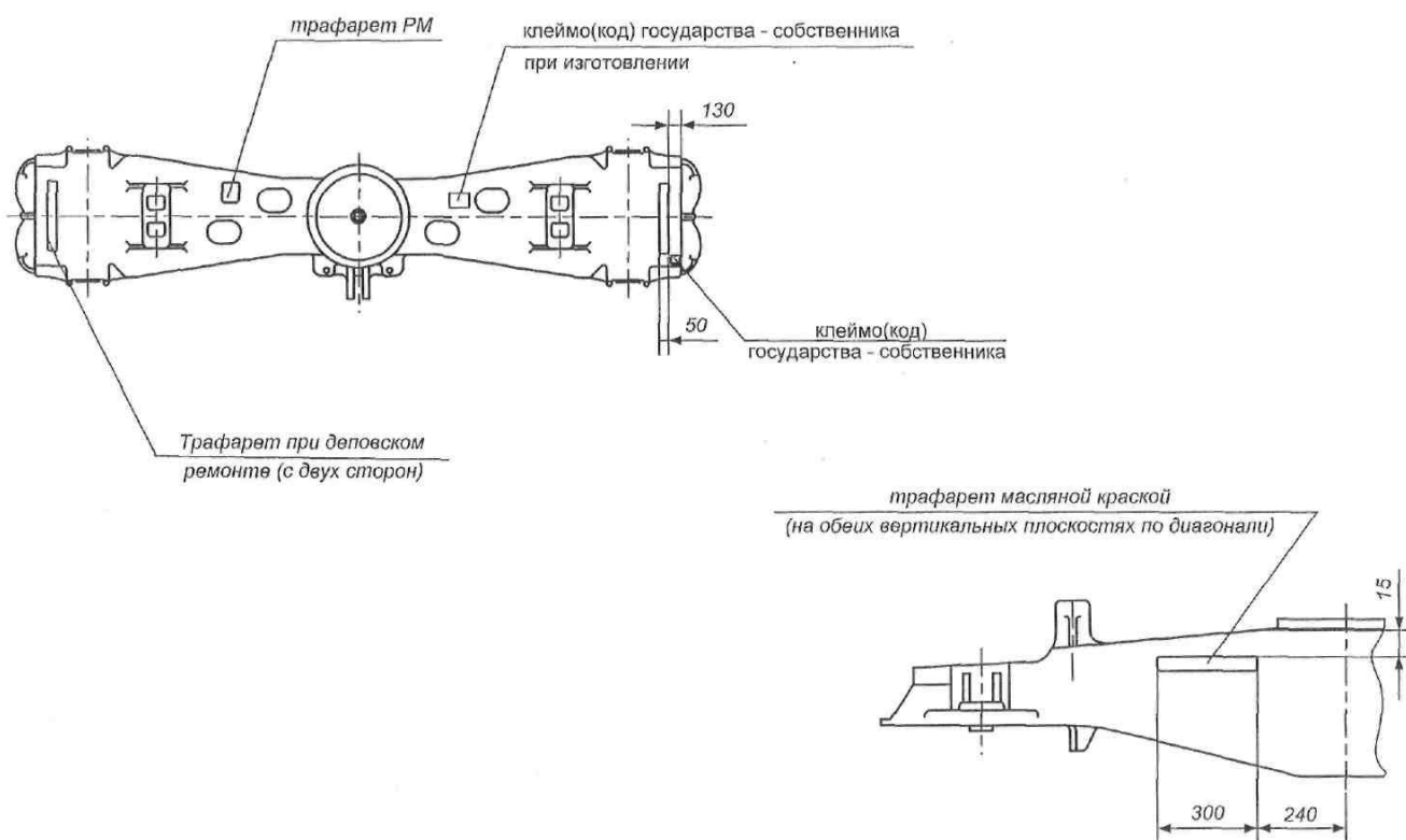
Рисунок Б.3 Места нанесения трафаретов и клейм на надрессорной балке
