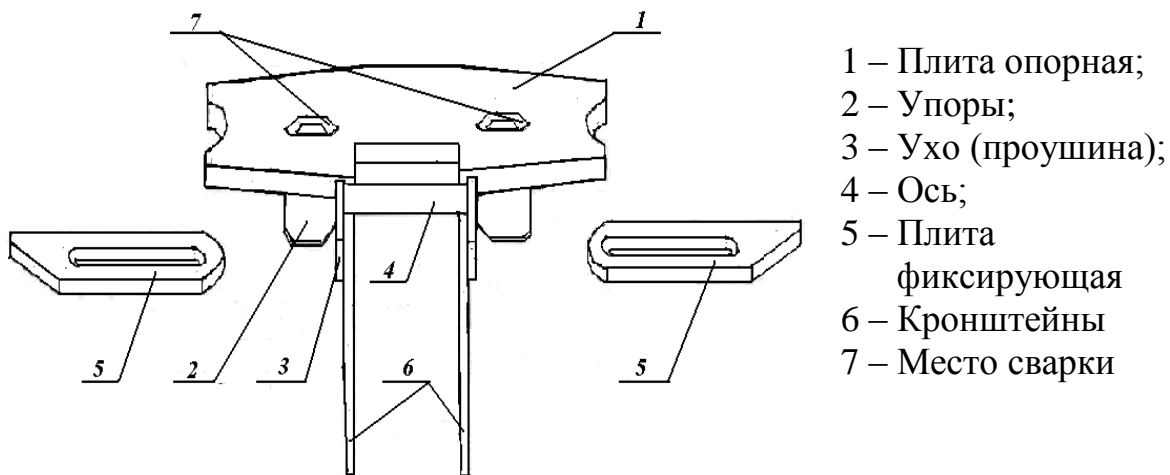
Рисунок 22. Плита с двумя упорами 31883-НСБ (нерабочее положение).
