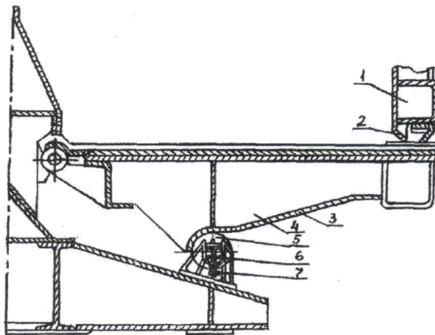
Рисунок 5 - Расположение крышки разгрузочного люка
