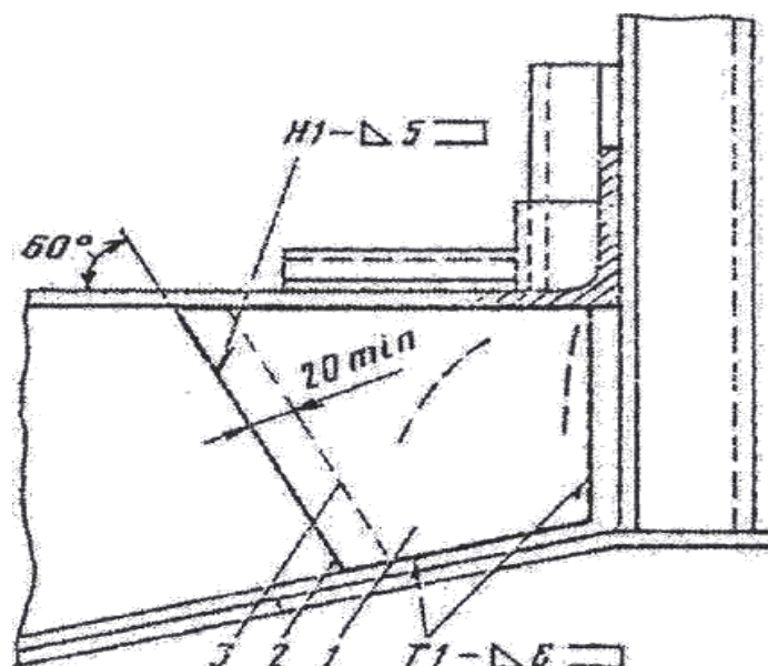
Рисунок 7 - Отремонтированный вертикальный лист промежуточной балки
