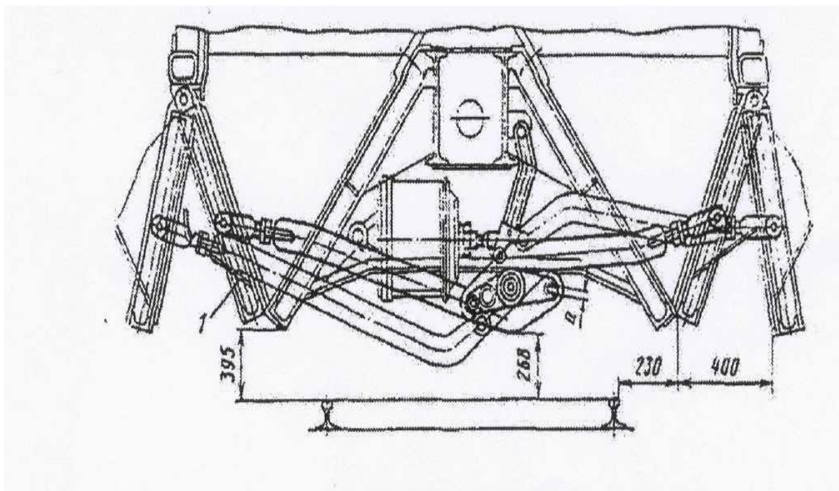
Рисунок 9 - Механизм разгрузки
