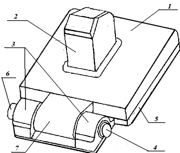
Рисунок 19. Плита опорная с упором литая 31896-НСБ (рабочее положение)
