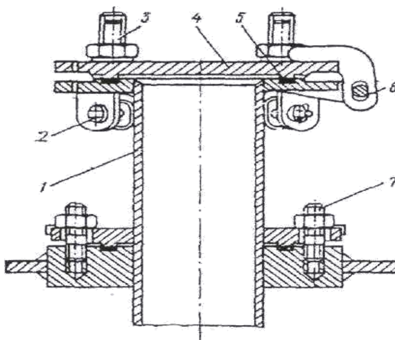
Рисунок 16 Сливное устройство
