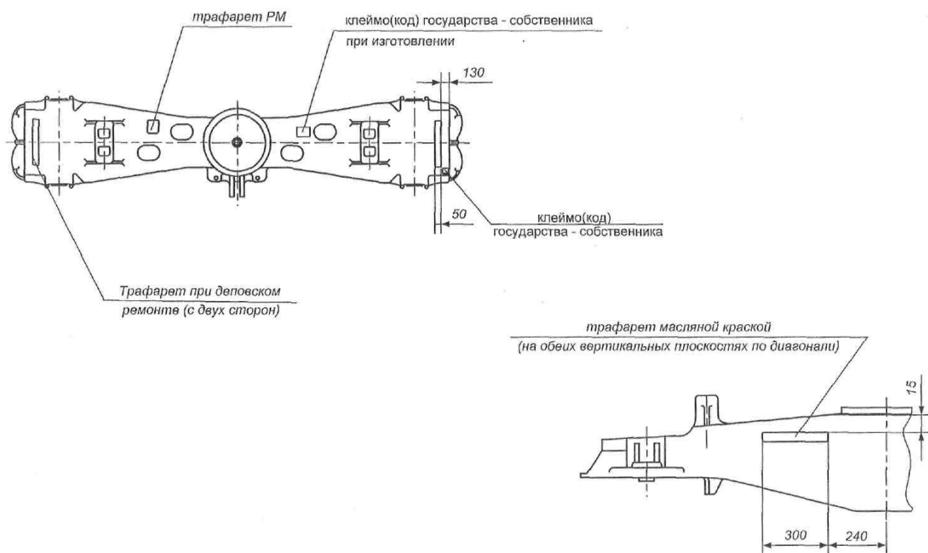
Рисунок Б.3 Места нанесения трафаретов и клейм на наддрессорной балке
