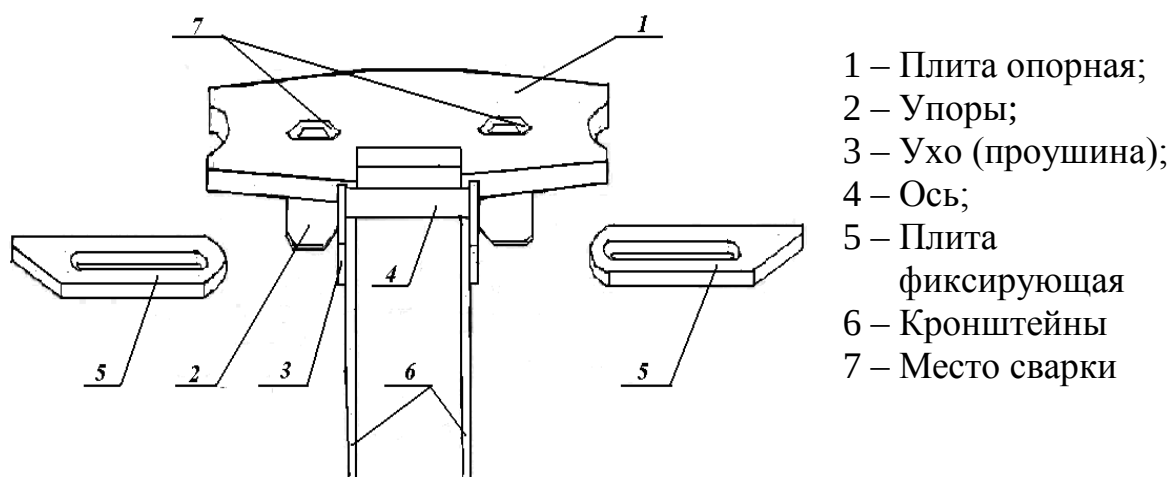
Рисунок 22. Плита с двумя упорами 31883-НСБ (нерабочее положение).
