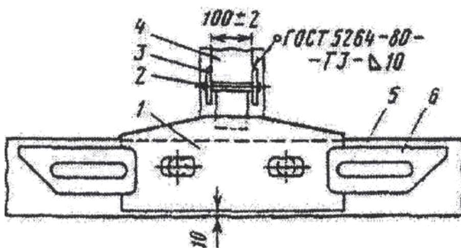
Рисунок 15 Опорная плита с упорами
